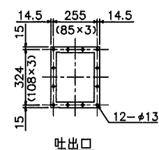
吐出口
