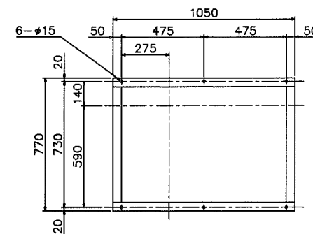
基礎寸法
