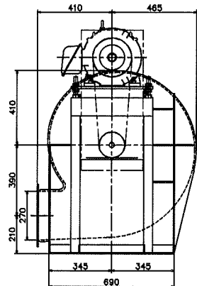
右回転下部水平
