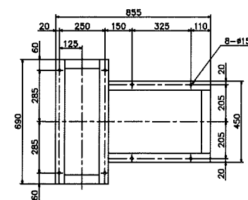
基礎寸法
