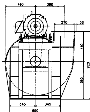
左回転上部垂直
