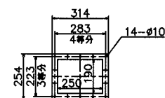
吐出口
