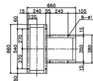
基礎穴寸法
