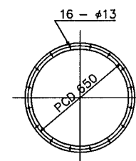
吸込口
