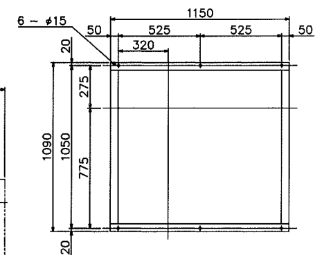
基礎寸法
